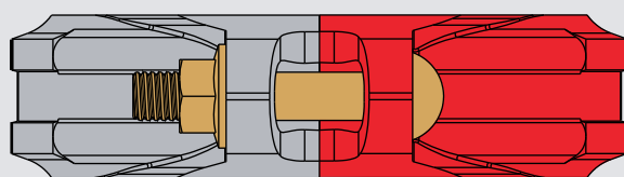
Das Gradsitzdesign der PicoFix Rohrkupplung Typ 901 ermöglicht den Ausgleich von Ungenauigkeiten
