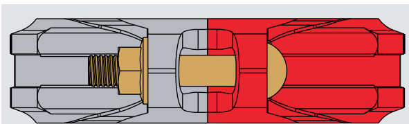
Das Gradsitzdesign der PicoFix Rohrkupplung Typ 901 ermöglicht den Ausgleich von Ungenauigkeiten
