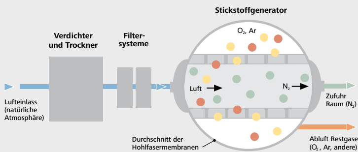
Systemschema zur Stickstoffherzeugung (Membran-Technologie)
