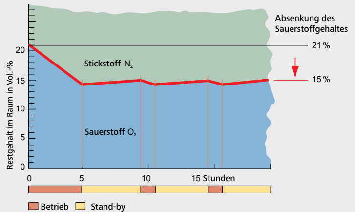
Betriebsphasen des Oxexo Prevent Brandvermeidungssystems
